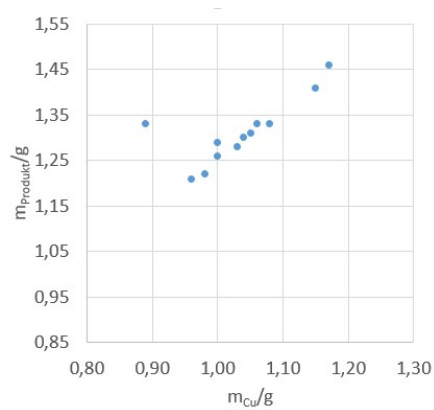
Abbildung 2. Gegenüberstellung der gemessenen Massen der Kupferplättchen und der Reaktionsprodukte.
